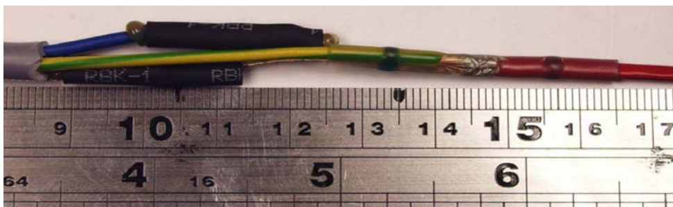
Figure 2 – Réalisation de la jonction froide en usine
