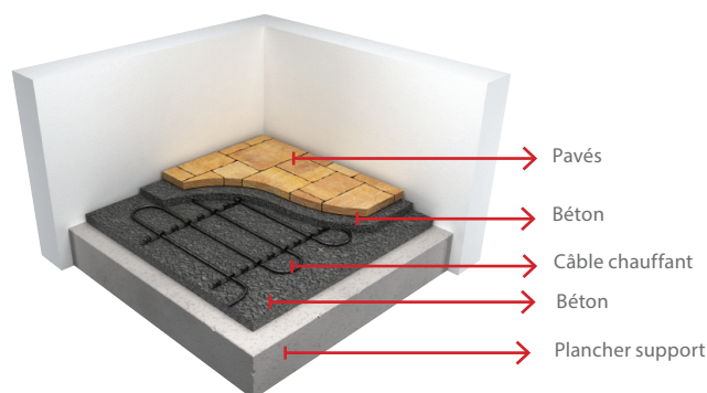
Câble à installer sous pavés
