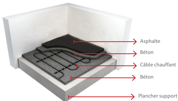
Câble à installer sous asphalte
