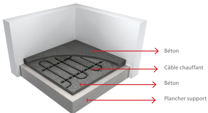
Câble à installer sous béton
